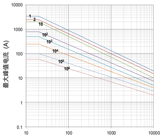
脉冲持续时间 (μs) SFV10D820KT to SFV10D122KT
